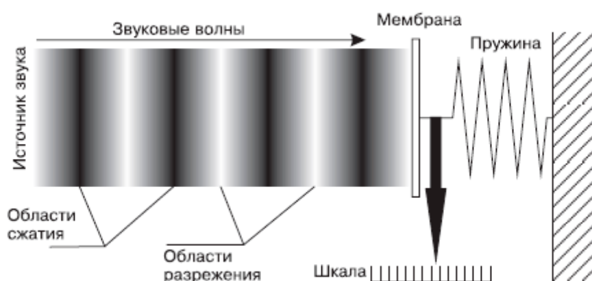
Рис. 1.1. Звуковые волны и звуковое давление
