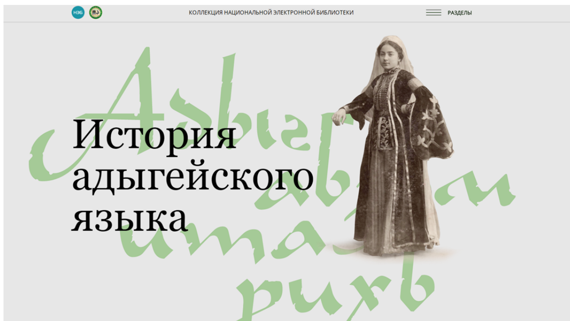
Рис. 1. Веб-страница проекта
