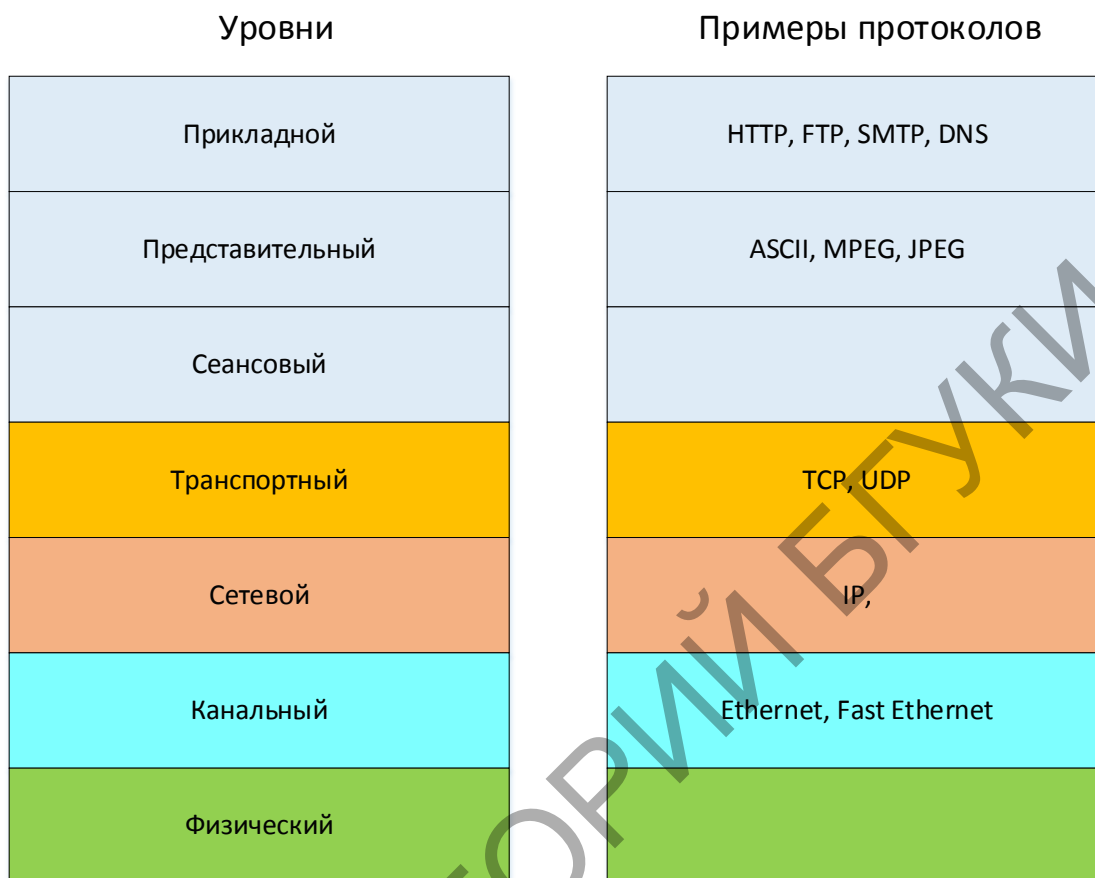
Рис. 9.3 – Примеры протоколов взаимодействия уровней
