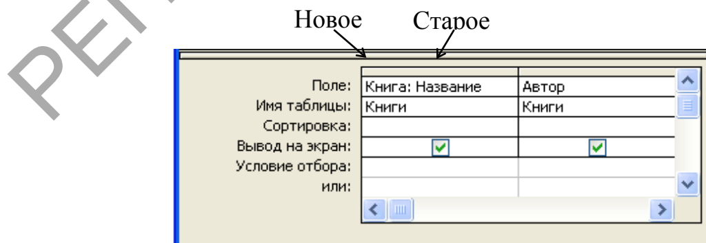
Рис. 3. Переименование поля.
