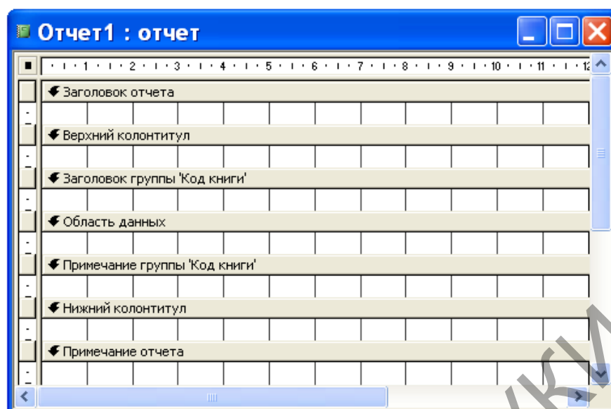
Рис. 6. Макет отчета.
