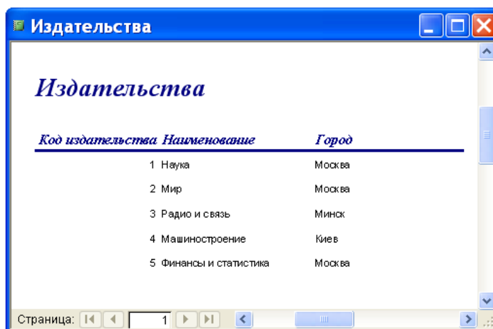
Рис. 4. Автоотчет ленточный.
